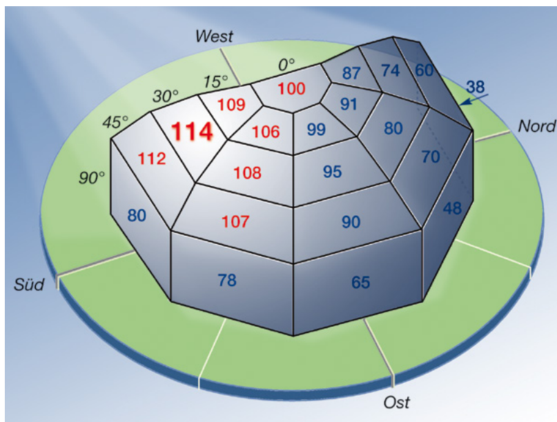
Abb. 3.4: Angaben zur solaren Einstrahlung in Prozent in Abhängigkeit von Ausrichtung und Neigung der Flächen (Zeichnung: Darja Süßbier, verändert nach: Weller et al. 2009: 12)
